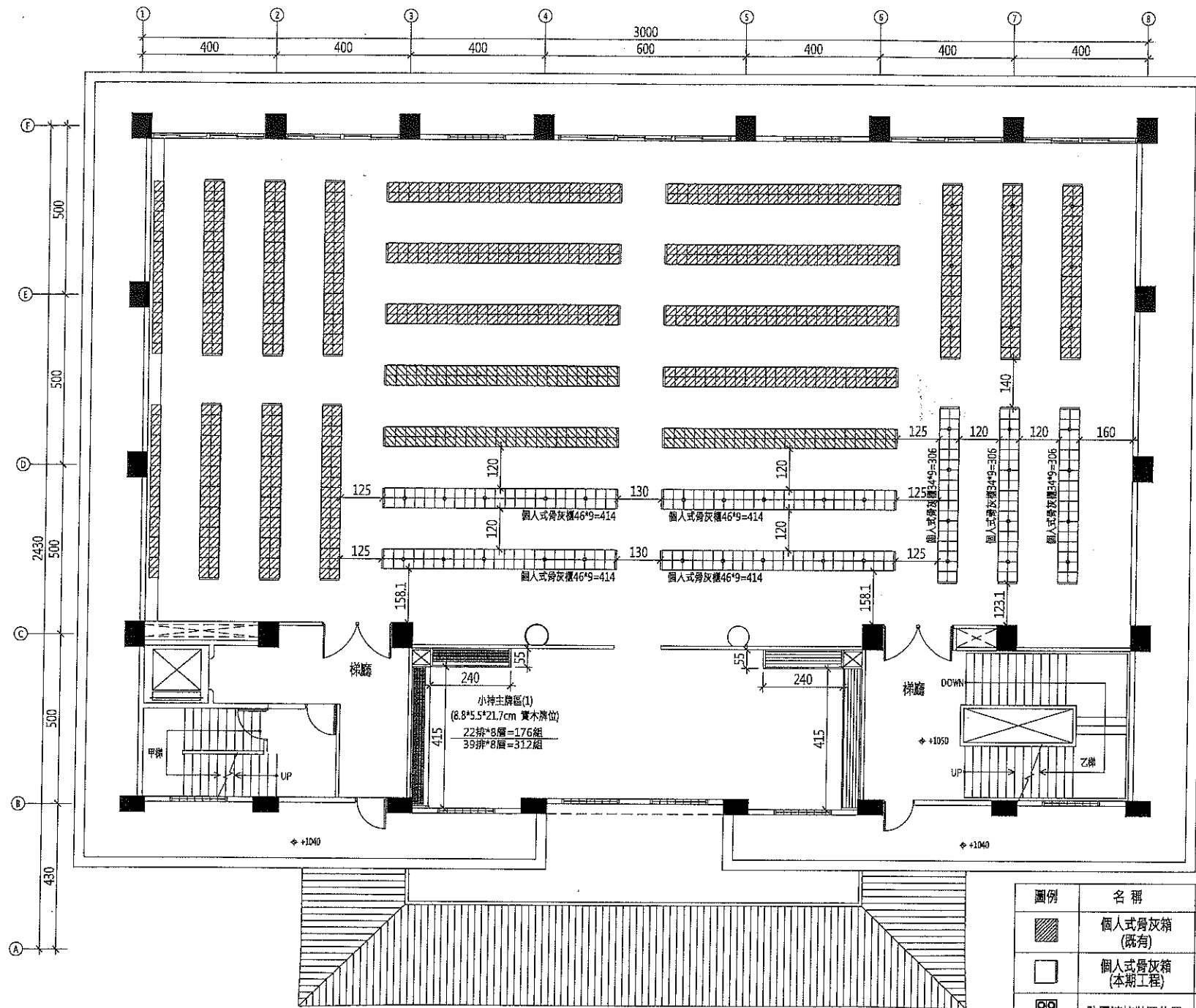
三層平面圖
