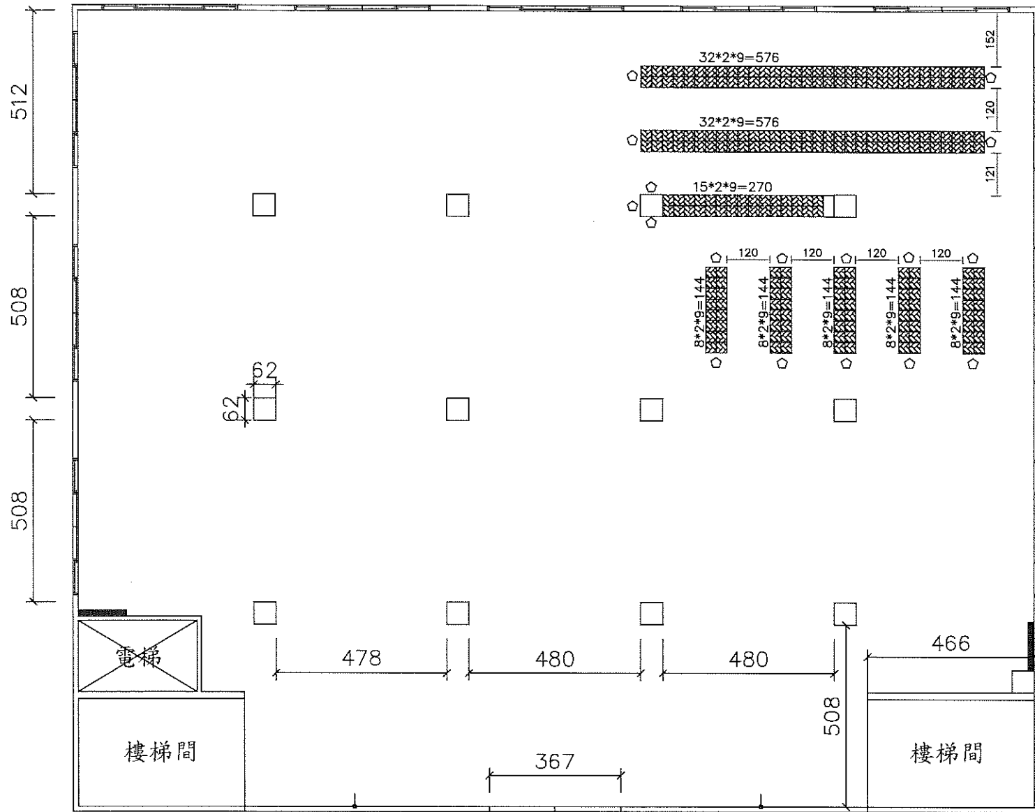
五樓平面圖
